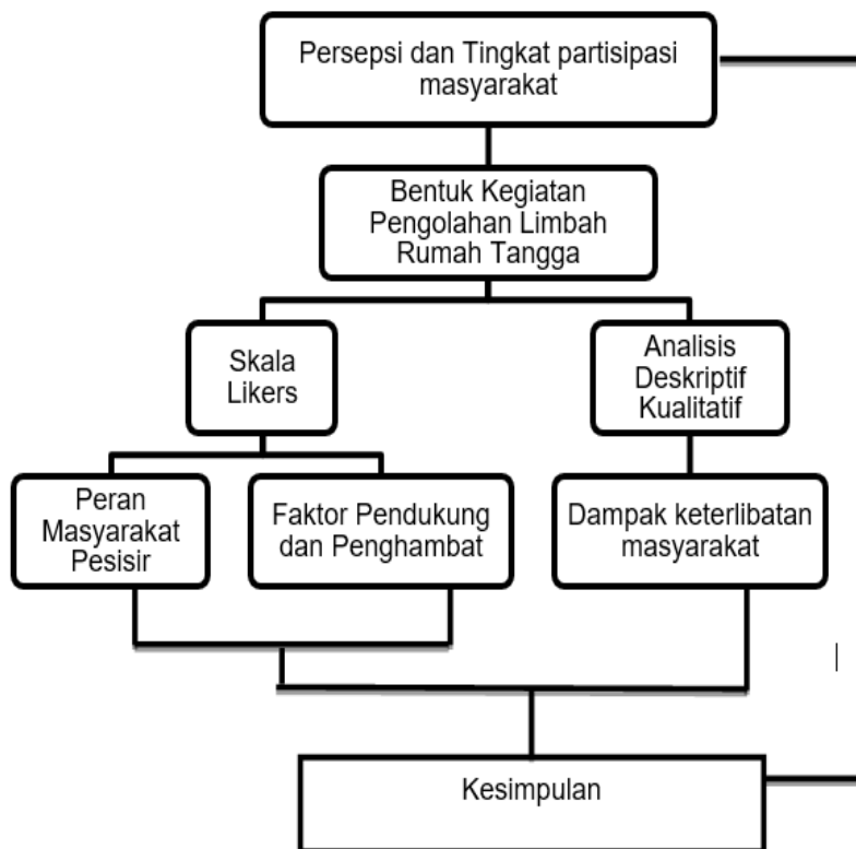
Gambar 1. Kerangka pikir
