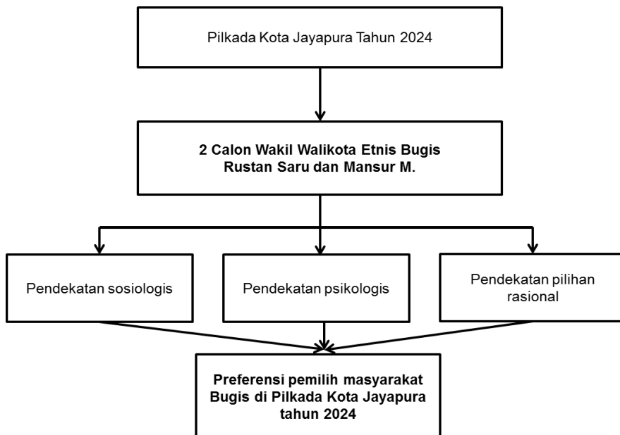
Gambar 1.2 Skema Berpikir
