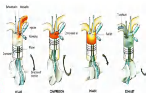
gambar 3. Siklus kerja motor diesel 4 langkah Sumber : (Centre, 2016)
