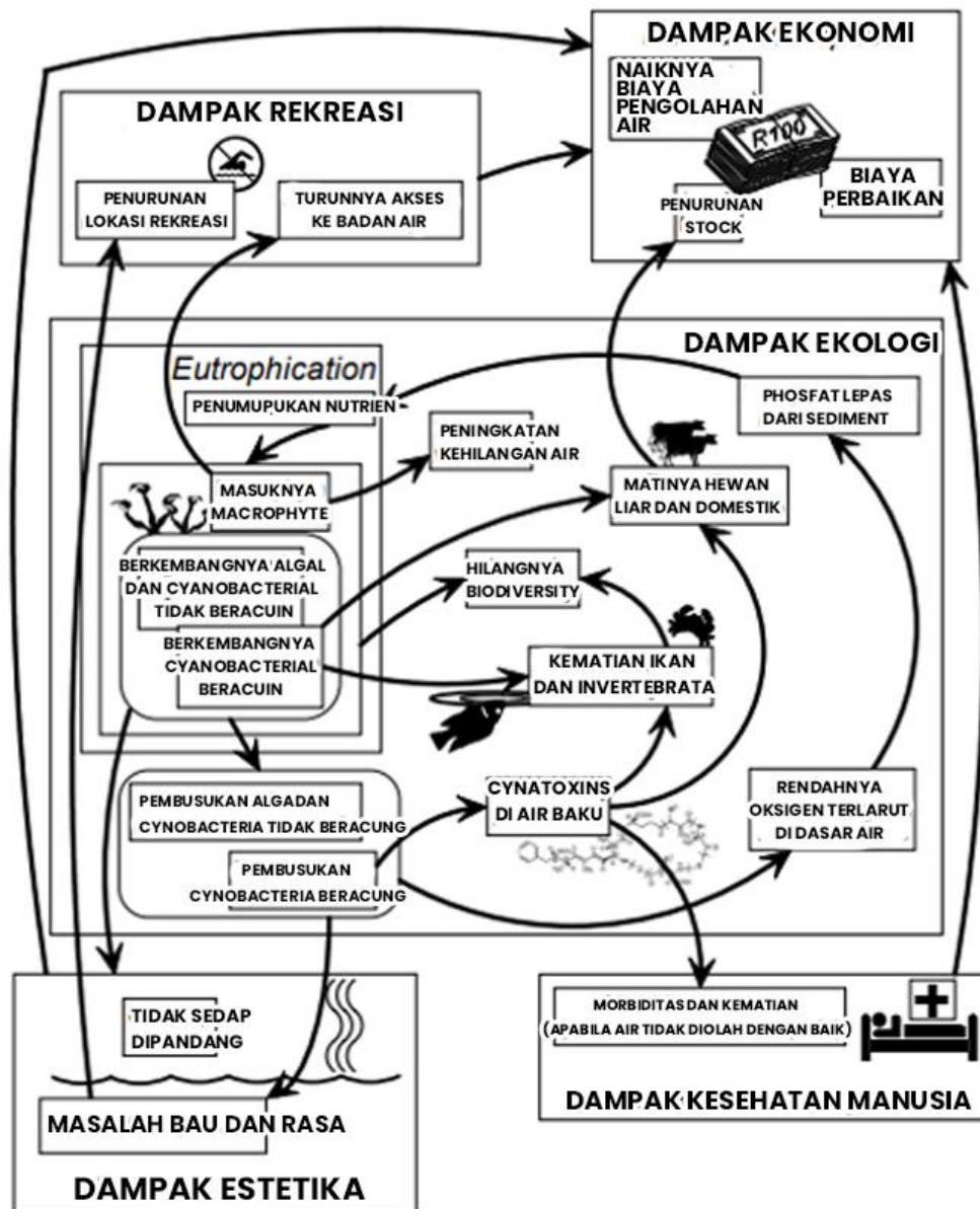
Gambar 5 Dampak spesifik eutrofikasi Sumber: (Ngatia & Taylor, 2019)
