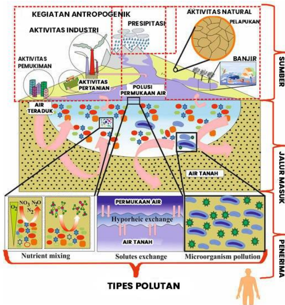
Gambar 1 Diagram skematik pencemaran di perairan.
