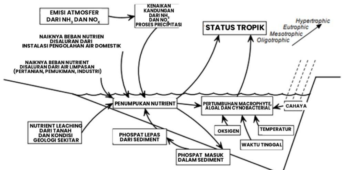
Gambar 4 Ilustrasi sederhana faktor terjadinya eutrofikasi
