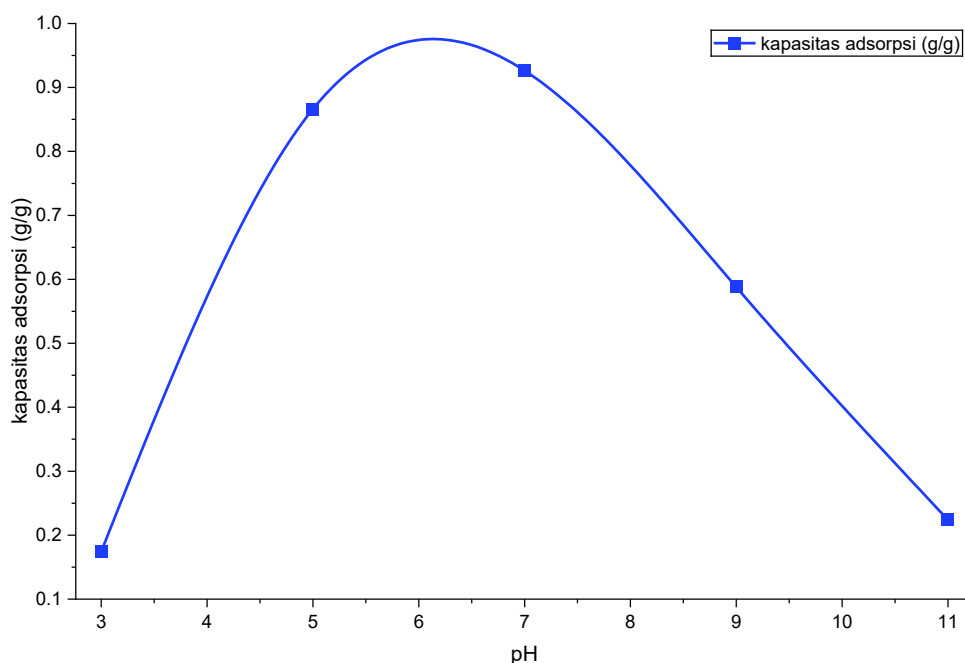
Gambar 3.5 Grafik variasi pH dengan jumlah minyak yang teradsorpsi oleh aerogel selulosa
