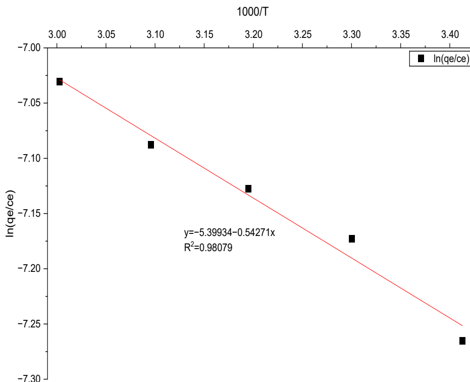
Gambar 3.11 Grafik \ln K terhadap 1000/T untuk memperkirakan parameter termodinamika adsorpsi minyak ke dalam aerogel
