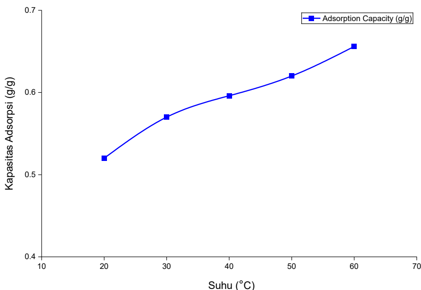
Gambar 3.6 Grafik pengaruh variasi suhu terhadap adsorpsi minyak aerogel Selulosa
