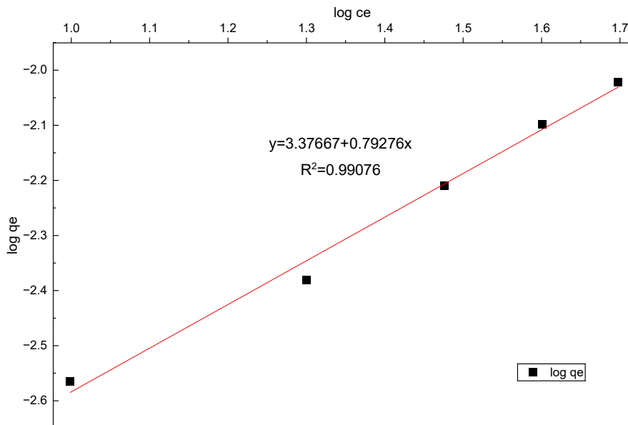
Gambar 3.9 Grafik isoterm Freundlich adsorpsi minyak
