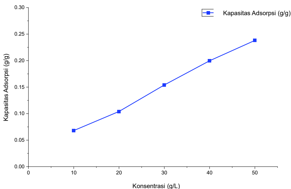
Gambar 3.7 Grafik pengaruh konsentrasi terhadap adsorpsi minyak oleh aerogel selulosa
