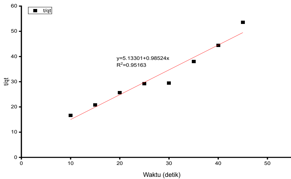
Gambar 3.4 Grafik kinetika orde dua semu adsorpsi minyak
