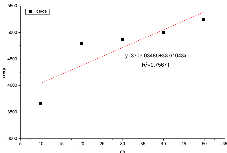
Gambar 3.8 Grafik isoterm Langmuir adsorpsi minyak
