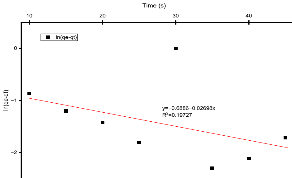
Gambar 3.3 Grafik kinetika orde satu semu adsorpsi minyak
