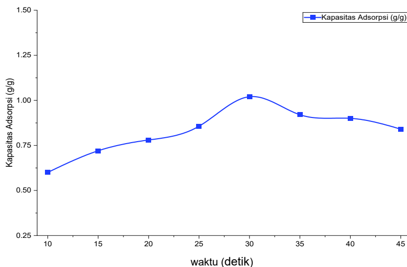
Gambar 3.1 Grafik variasi waktu kontak dengan jumlah minyak yang teradsorpsi oleh aerogel selulosa
