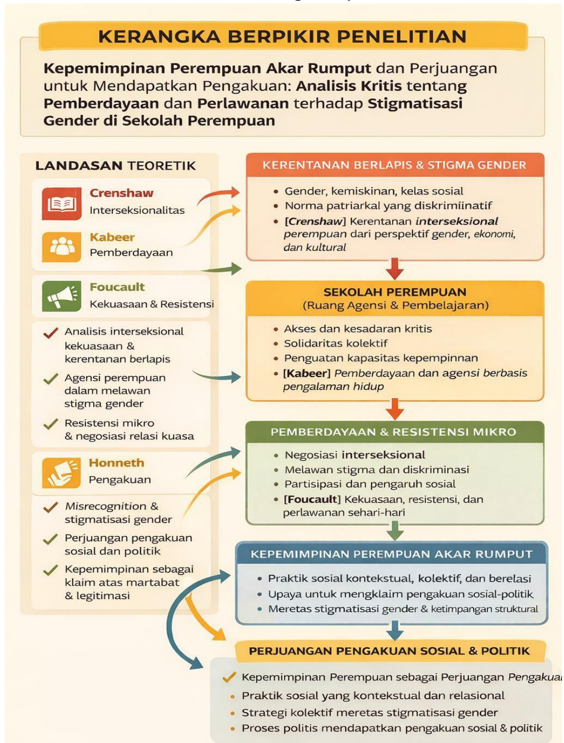
Gambar 2. Kerangka Berpikir
