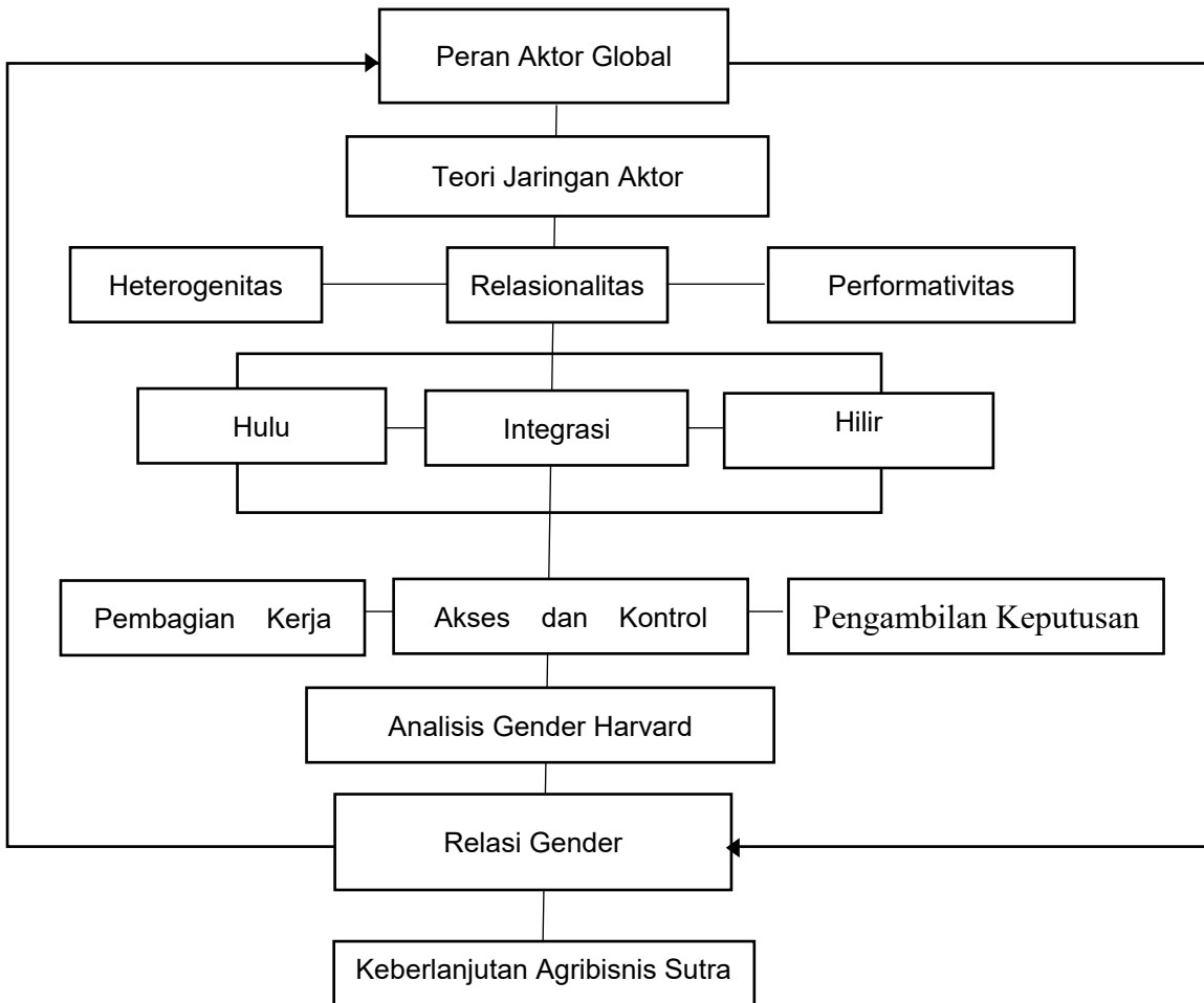
Gambar 1. Kerangka Pemikiran
