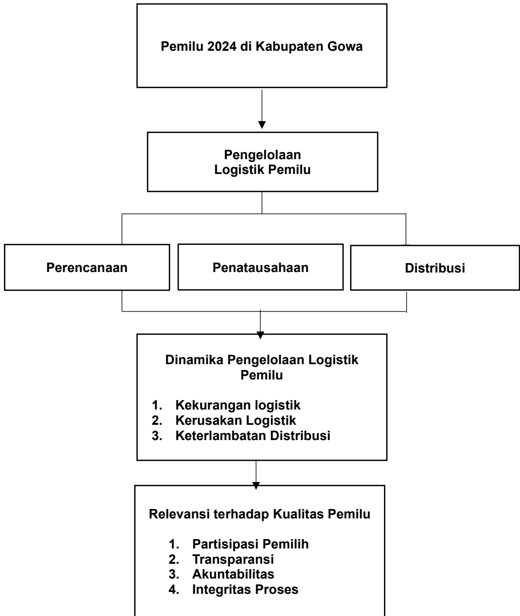
Gambar 1 Skema Pemikiran
