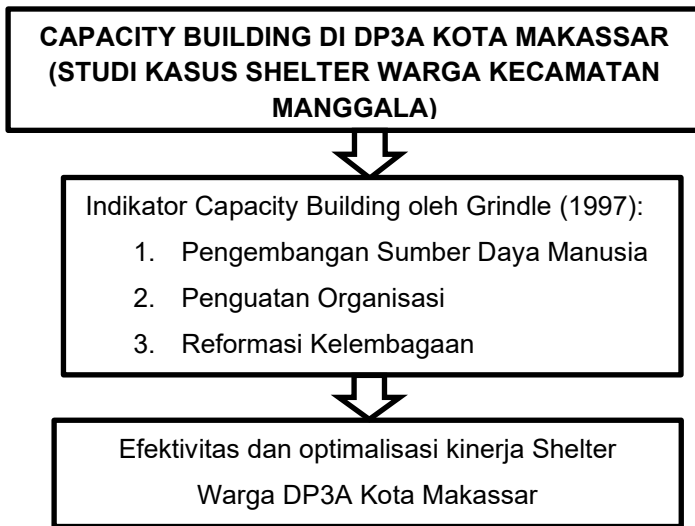
Gambar 2 Kerangka Pikir
