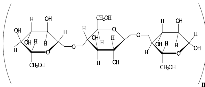
Gambar 1 . Struktur selulosa
