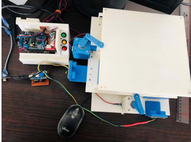
a. alat uji shake table
