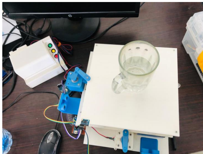
d. Pengujian shake table 2
