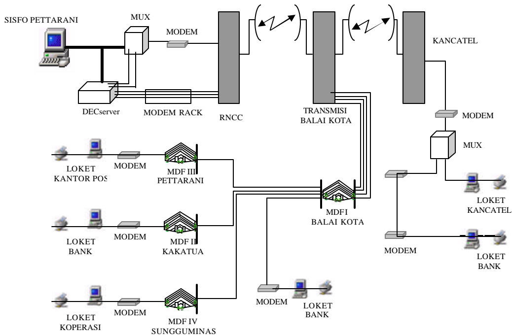
Gambar 2. Konfigurasi SOPP
