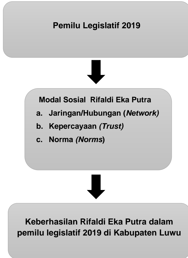
Gambar 1. Skema Penelitian
