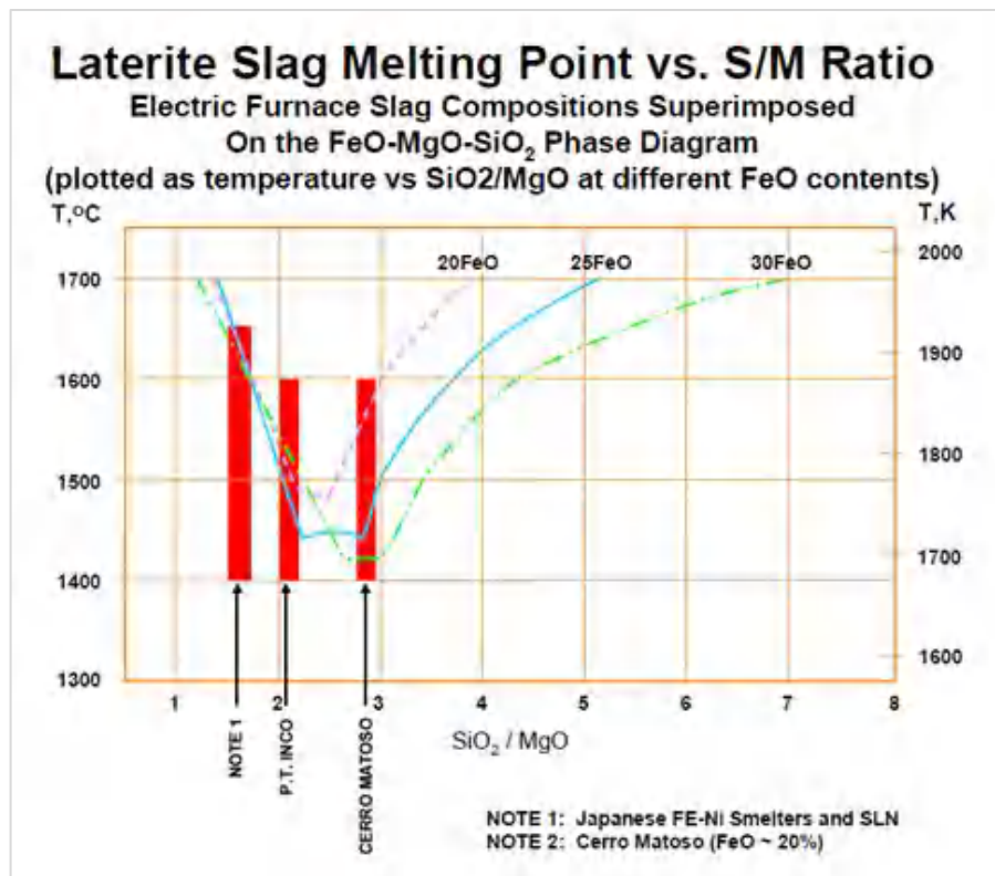
Gambar 10 Titik leleh slag vs rasio \text{SiO}_2/\text{MgO} (Dalvi et al. , 2004)
