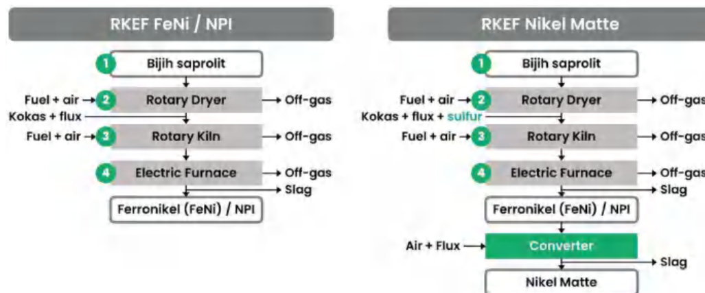
Gambar 9 Diagram alir peleburan dengan metode RKEF (Pintowantoro & Abdul, 2019)
