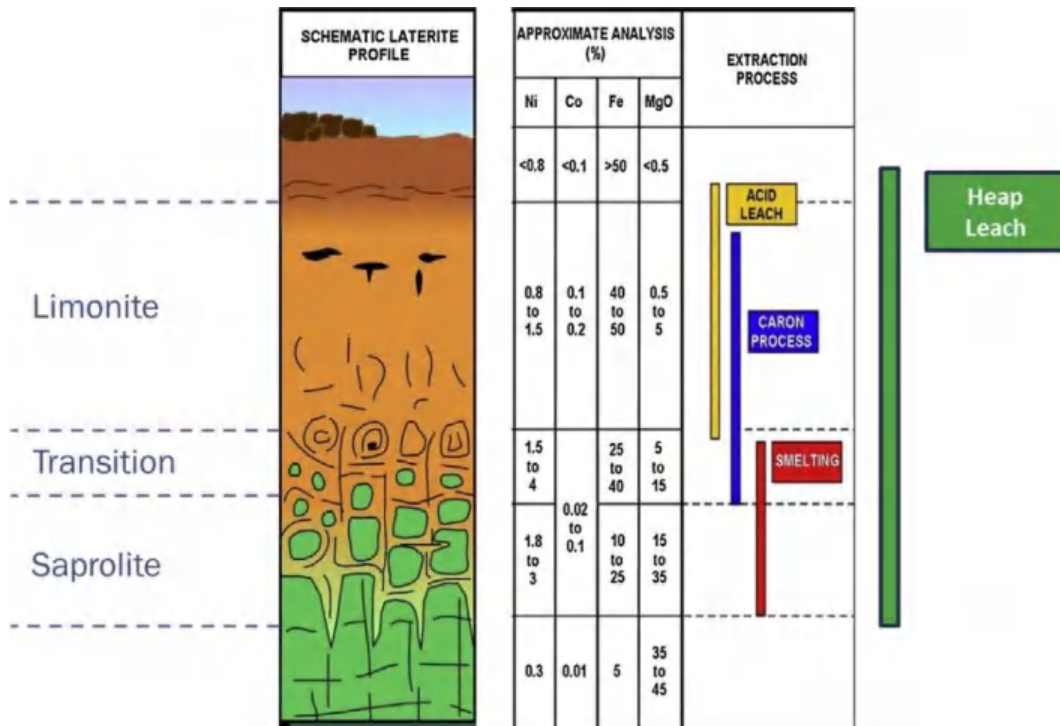
Gambar 11 Opsi pemrosesan untuk laterit nikel (Brand et al. , 1998)
