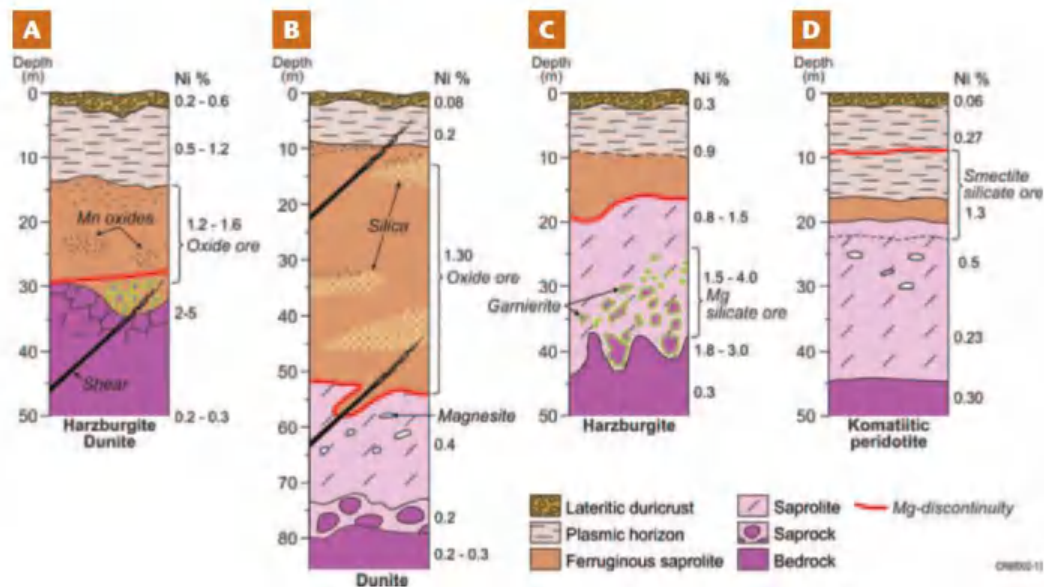
Gambar 4 Profil laterit yang terbentuk pada batuan ultramafik terserpentinisasi menunjukkan bijih nikel laterit utama. (A) oxide ; (B) partly silicified oxide ; (C) hydrous Mg silicate ; (D) Clay silicate ((Butt & Cluzel, 2013)
