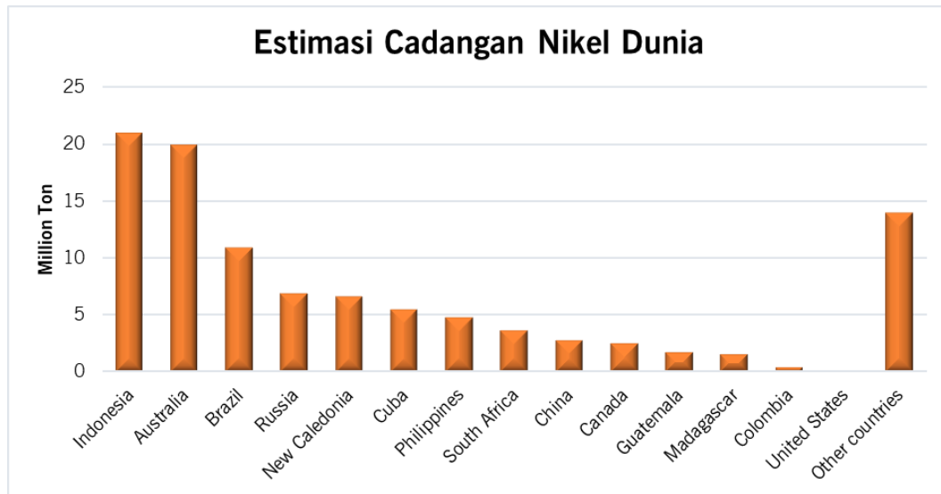
Gambar 7 Estimasi cadangan nikel dunia (USGS, 2020)
