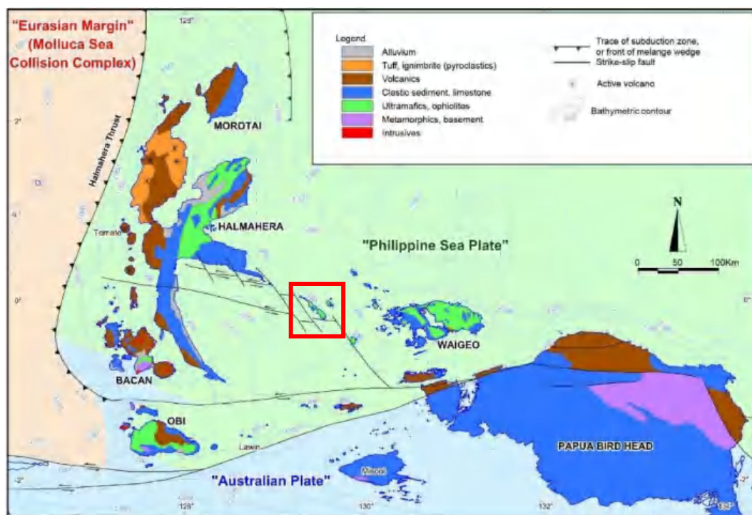
Gambar 1 Tektonik dan geologi Halmahera - wilayah Kepala Burung Papua (Prihatmoko et al. , 2013). Lokasi penelitian ditunjukkan oleh blok berwarna merah
