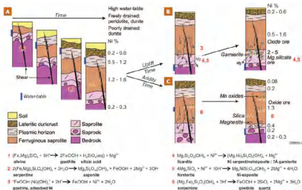
Gambar 3 Pembentukan dan evolusi endapan oksida ( oxide ) dan hydrous Mg silicate deposits . (A) Perkembangan progresif regolith laterit yang berdiferensiasi bawah iklim sabana yang lembab secara musiman di daerah dengan relief dan tektonik yang stabil. (B) Dengan pengangkatan dan di bawah iklim ama, pelindian dan reaksi/pertukaran Ni menghasilkan silikat Mg yangandung air. (C) Profil dimodifikasi selama perubahan ke iklim kering, dengan presipitasi magnesit dan silika (Butt & Cluzel, 2013)
