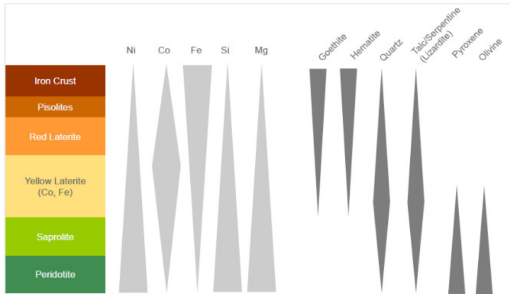
Gambar 6 Hubungan antara mineral dan kimia pada profil laterit silikat Mg-Si hidrat (König, 2021)
