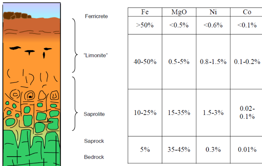
Gambar 5 Profil nikel laterit secara umum (Elias, 2002)
