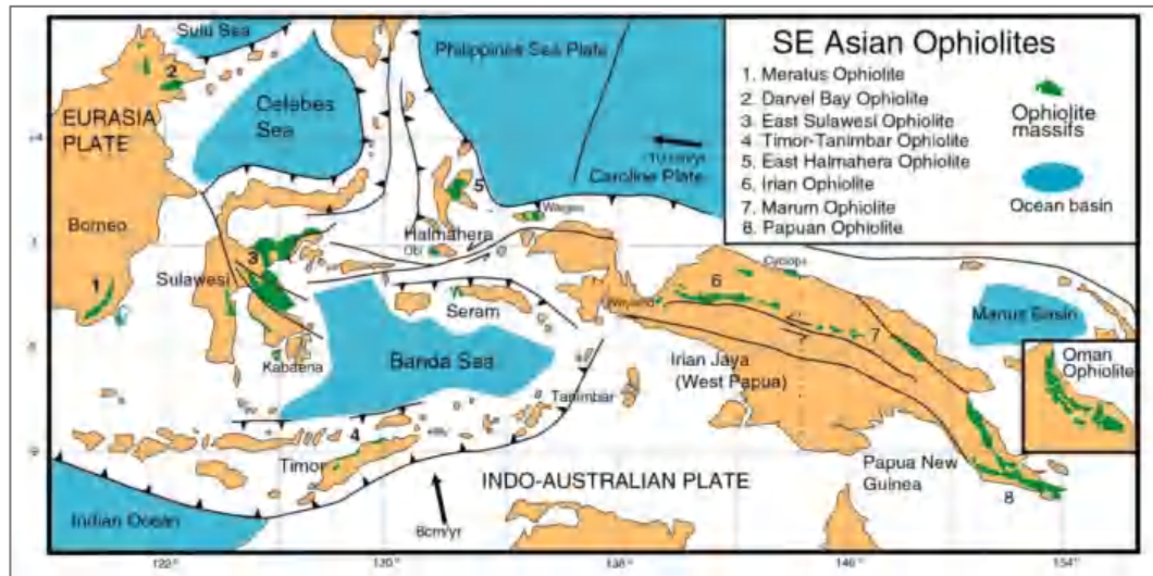
Gambar 8 Sebaran ofiolit di kawasan timur Indonesia (Kadarusman, 2013)
