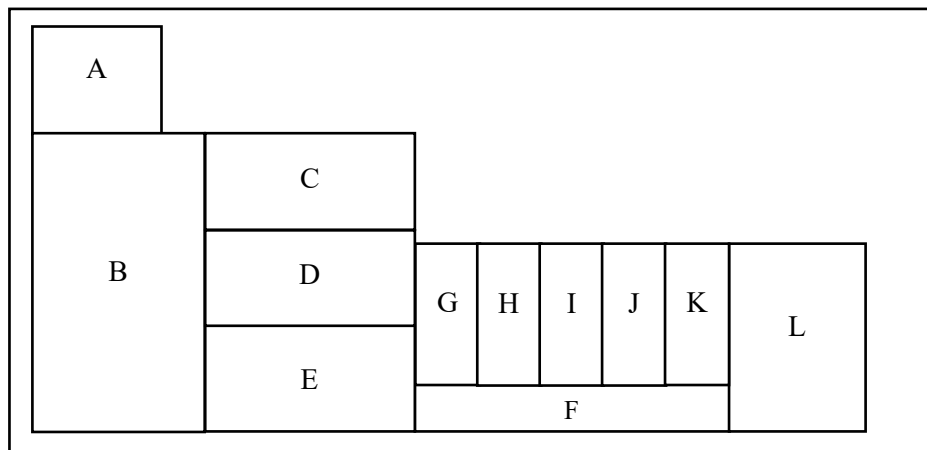
Gambar 4. Tata letak/layout kandang pemeliharaan kambing UD. Fadil Ternak
