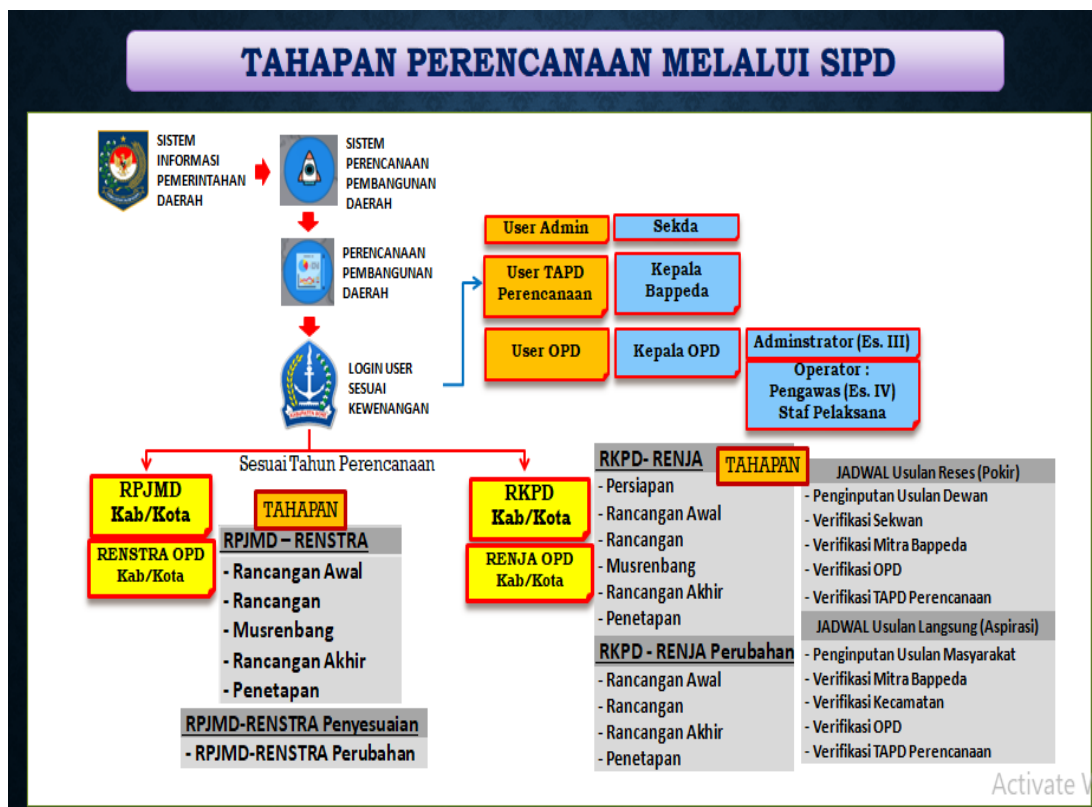
Tahapan Perencanaan Melalui Sistem Informasi Pemerintah Daerah Kabupaten Bone
