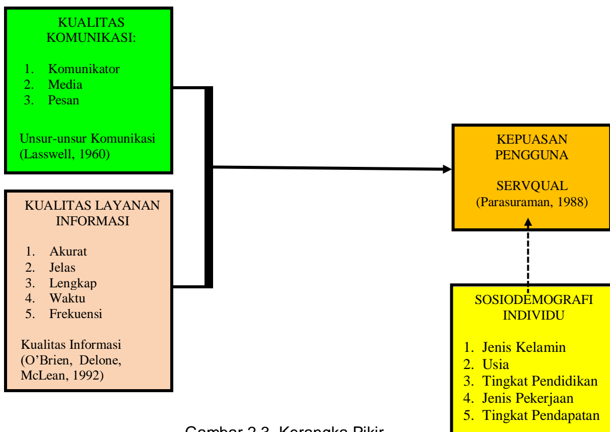
Gambar 2.3. Kerangka Pikir
