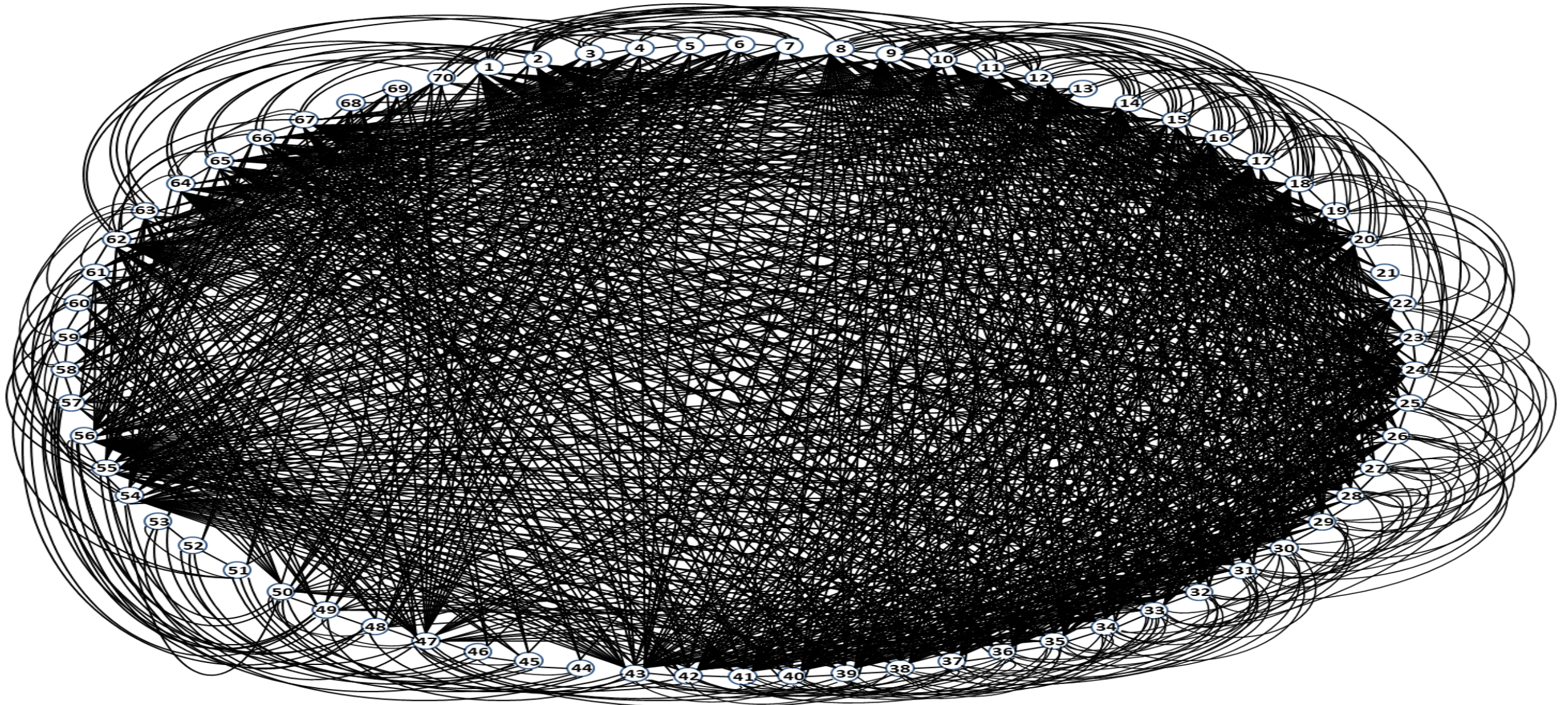
Lampiran 4. Representasi Graf Berbasis Interferensi Gelombang
