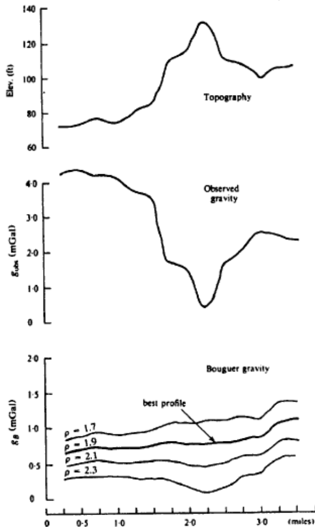
Gambar 2.19 Estimasi rapat massa dengan metode Nettleton (Telford et al., 1990)
