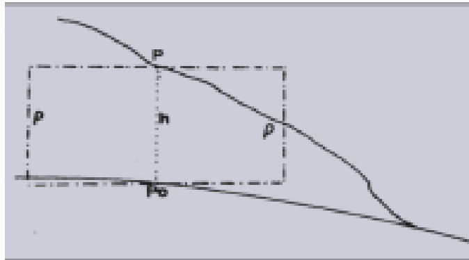
Gambar 2.15 Lempeng Bouguer dengan ketinggian h (Latifah, 2010)
