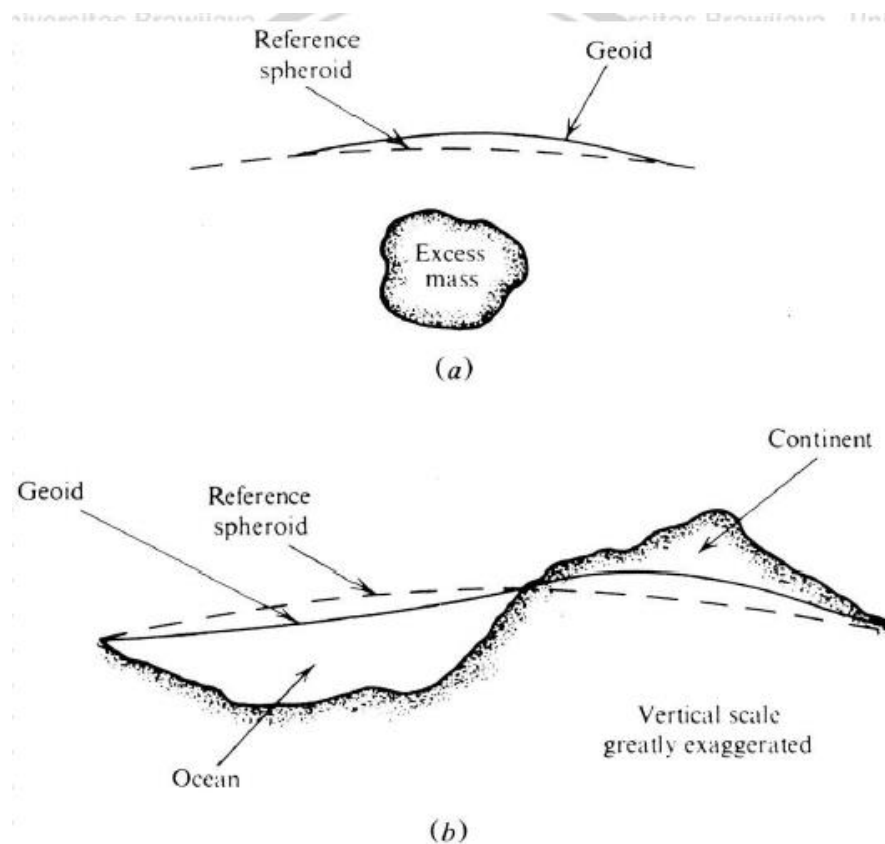
Gambar 2.10 Hubungan antara geoid, spheroid, topografi dan massa anomali (Telford et al., 1990)
