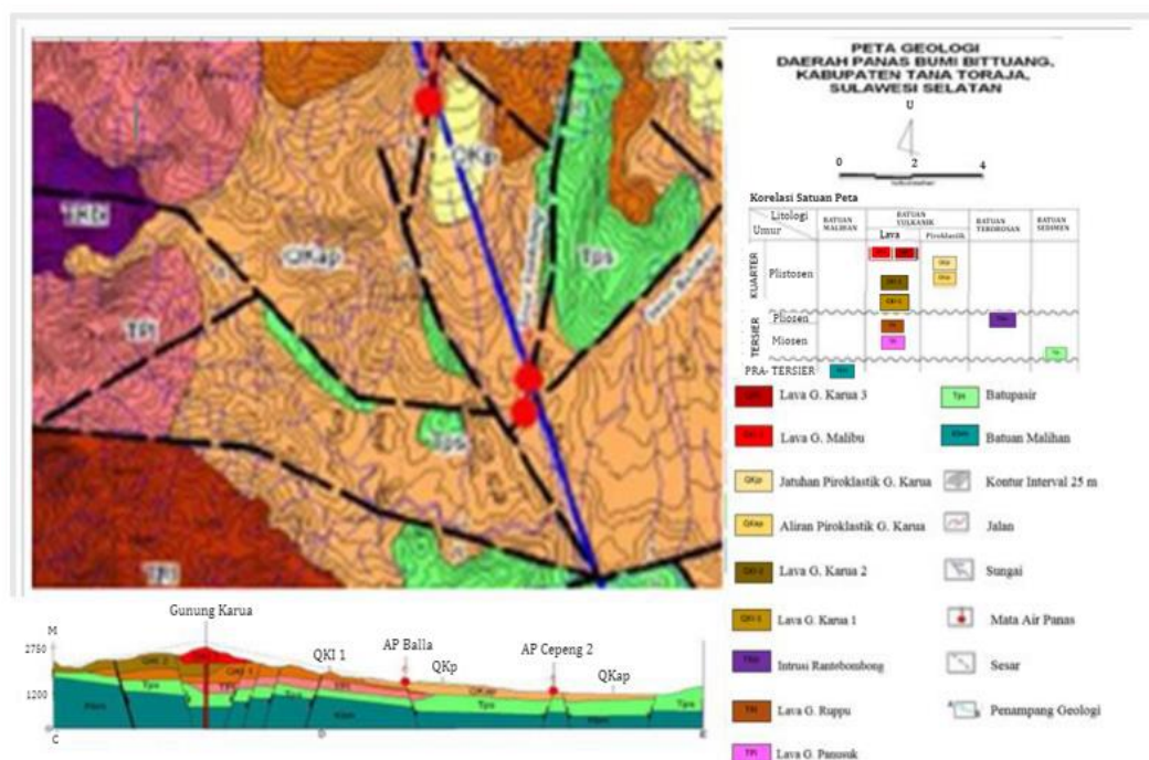
Gambar 2.2 Peta Geologi Daerah Panas Bumi Bittuang, Kab.Tana Toraja, Sulawesi Selatan(Soetoyo, 2010).
