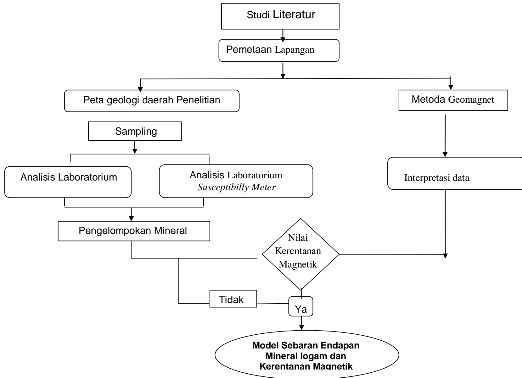
Gambar 1.1. Bagan alir sistematika penulisan dalam penentuan model sebaran endapan mineral logam
