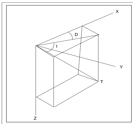
Gambar 2.2. Notasi unsur magnet sebagai vector medan magnet Bumi (Nettleton,1971 dalam Untung, M., 2001)
