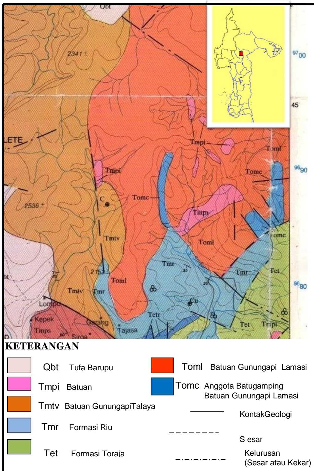
Gambar 2.1 Peta Geologi Regional Lembar Mamuju, Sulawesi ( Ratman, dan Atmawinta, 1993 ).
