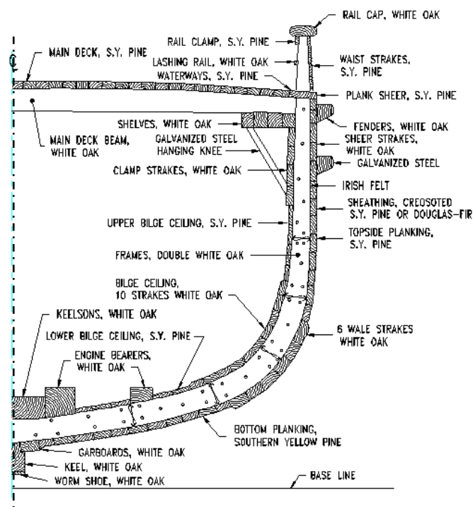
Gambar 8. Midship section dari salah satu Kapal Pelra
