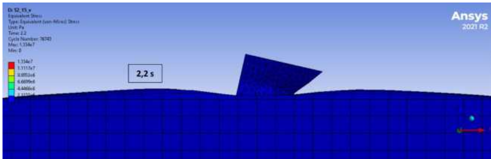
Lampiran 3. Data hasil simulasi drop test pada model haluan 2 (Sudut kemiringan linggi haluan 57 derajat)
