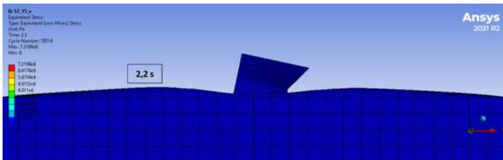
Lampiran 4. Data hasil simulasi drop test pada model haluan 3 (Sudut kemiringan linggi haluan 62 derajat)
