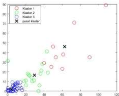
Klaster 4
