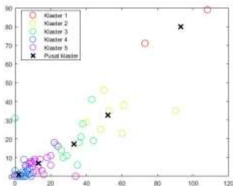
Klaster 5
