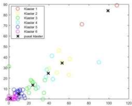
Klaster 7
