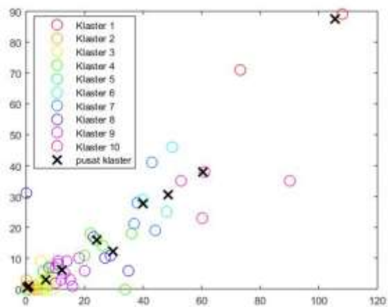
Klaster 10
