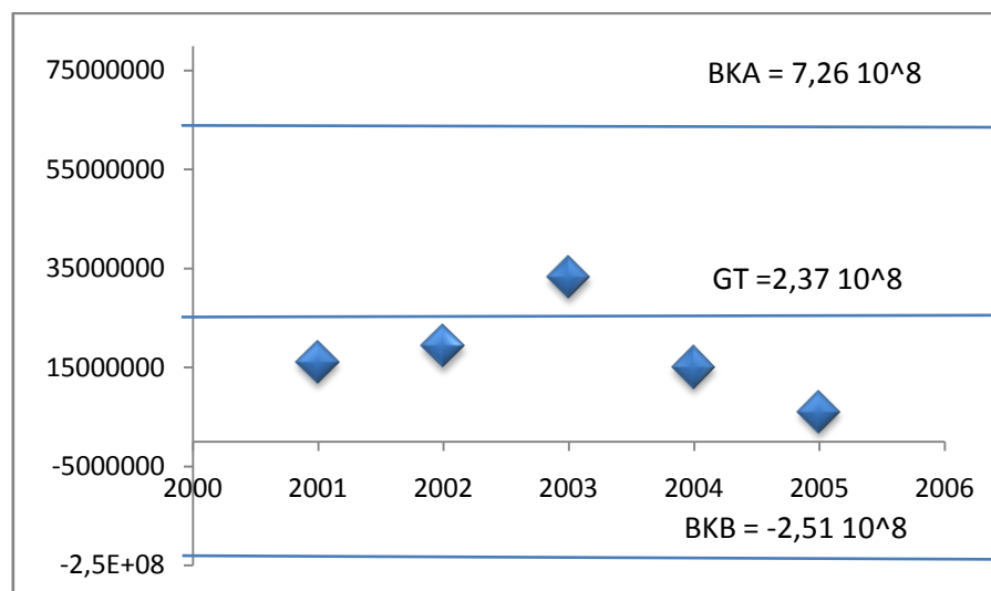
Gambar 4.2. Grafik bagan kendali Vektor Variansi pada data memonitoring cuaca di Kota Semarang
