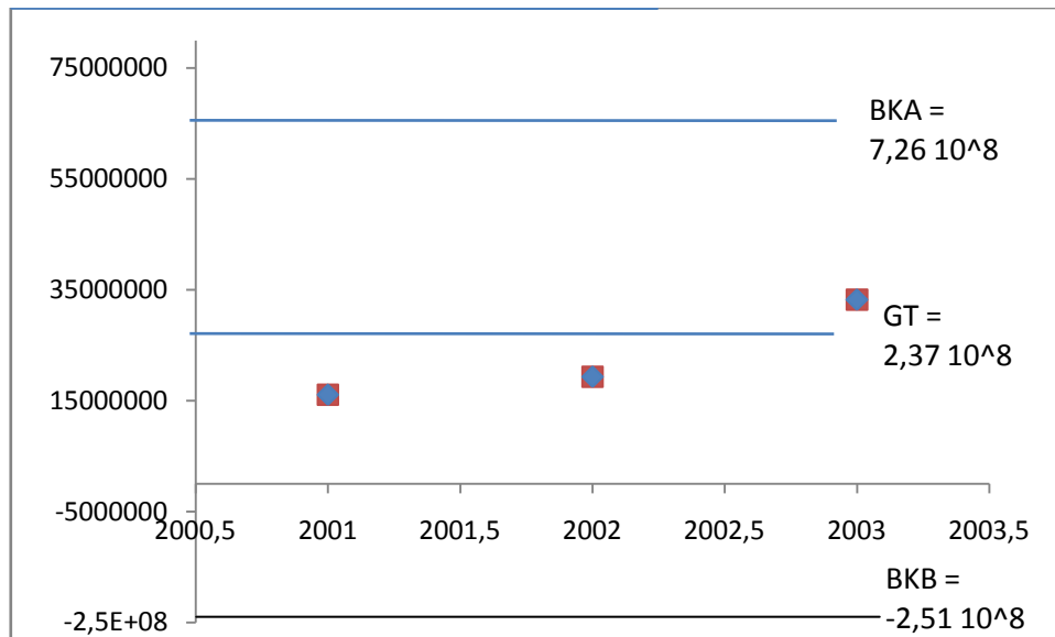
Gambar 4.1. Grafik bagan kendali Vektor Variansi pada data pendahuluan cuaca di Kota Semarang
