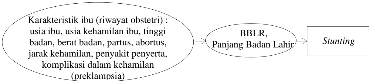
Gambar 3.1 Kerangka Konsep
