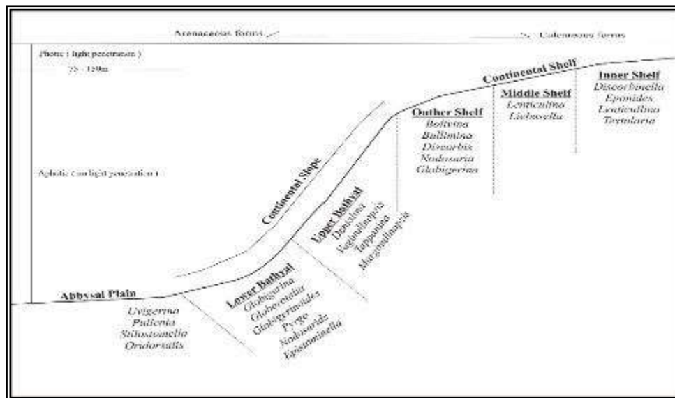
Gambar 2.2 Distribusi kandungan foraminifera bentonik dalam batuan sedimen dari paparan kontinen hingga abysal ( Haq dan Boersma (1980) dalam Pringgoprawiro, Kapid & Barmawidjaja, (1994)).
