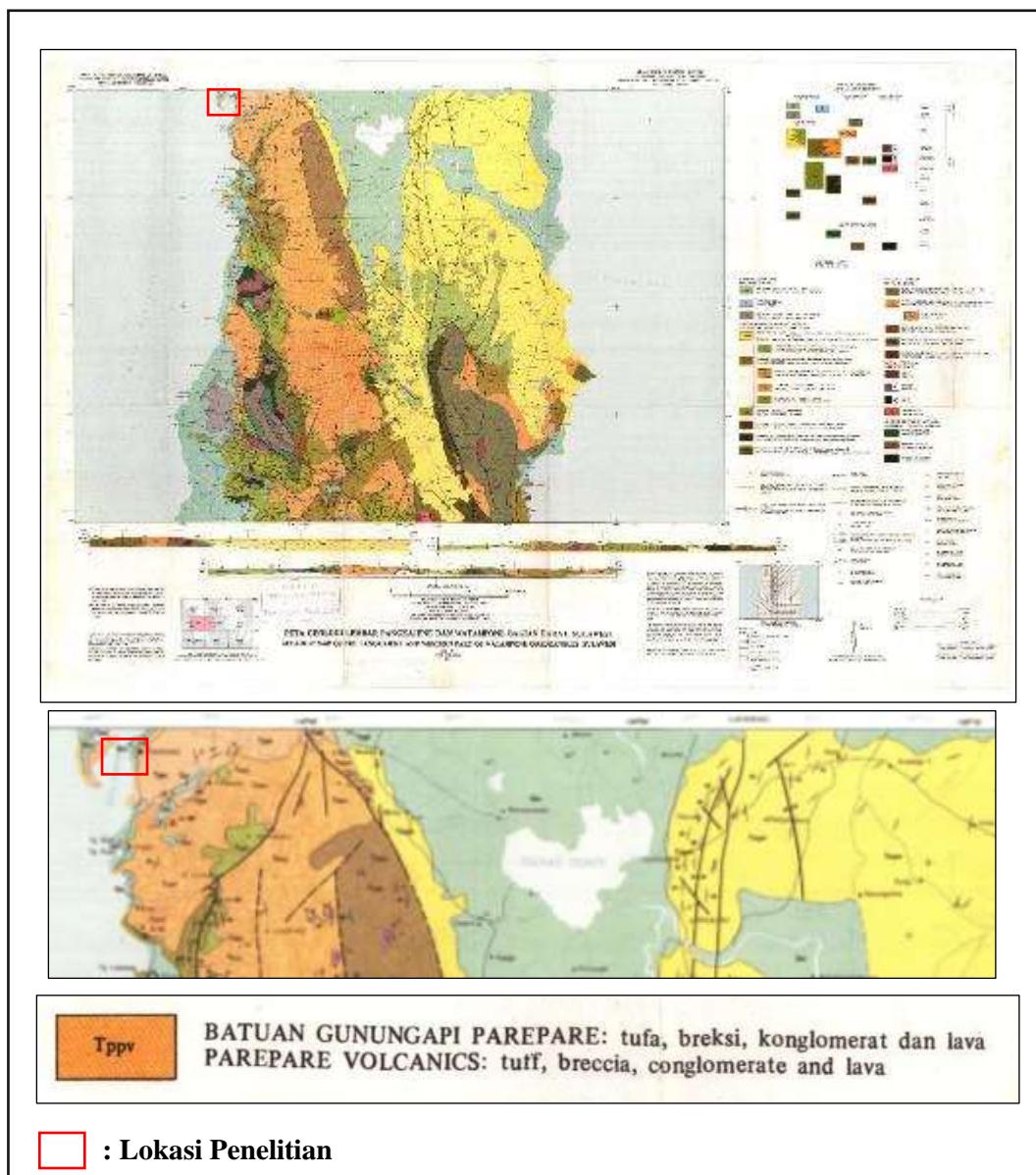
Gambar 2.1 Peta Geologi Regional Lembar Pangkajene dan Watampone Bagian Barat (Sukanto, 1982)
