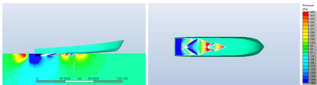
Gambar visualisasi static pressure pada model kapal tiga stepped V
