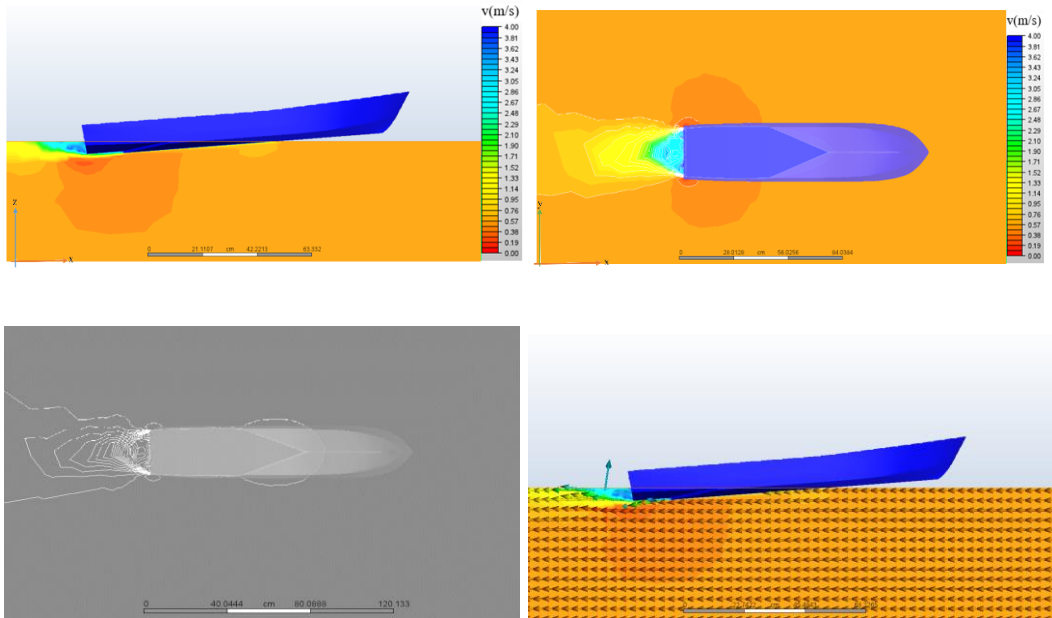
Gambar visualisasi velocity magnitude pada model kapal dua stepped V
