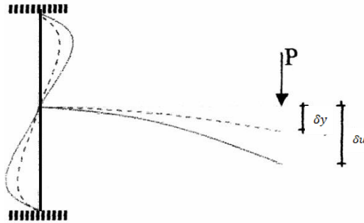
Gambar 5. Daktilitas Lendutan
