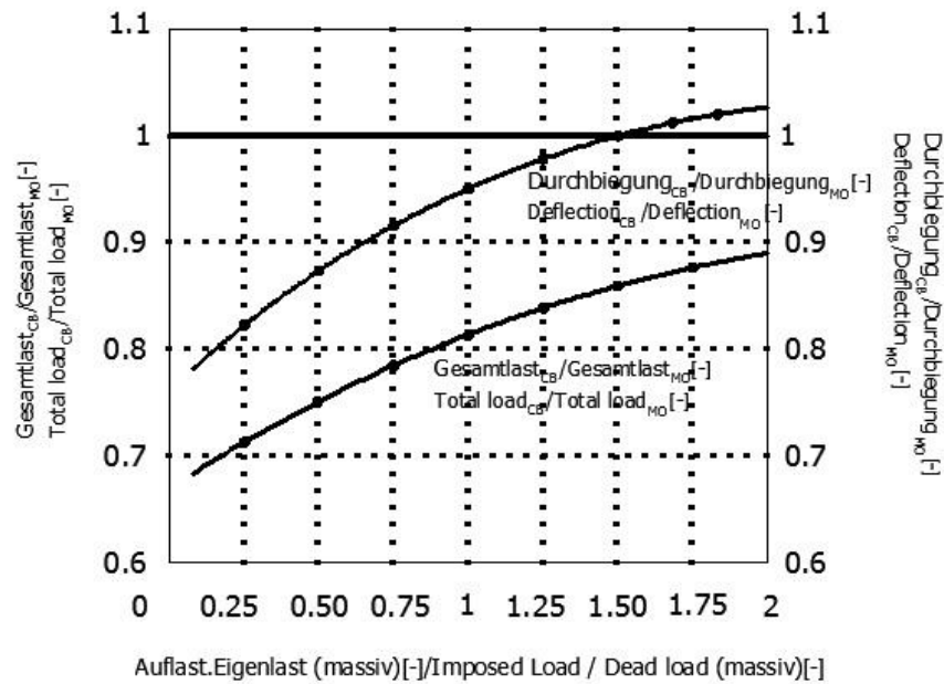
Gambar 14. Grafik Rasio Lendutan Pelat Beton Berongga Bola (CB) terhadap Pelat Beton Solid (MD) (Aldejohann dan Schnellenbach, 2005)
