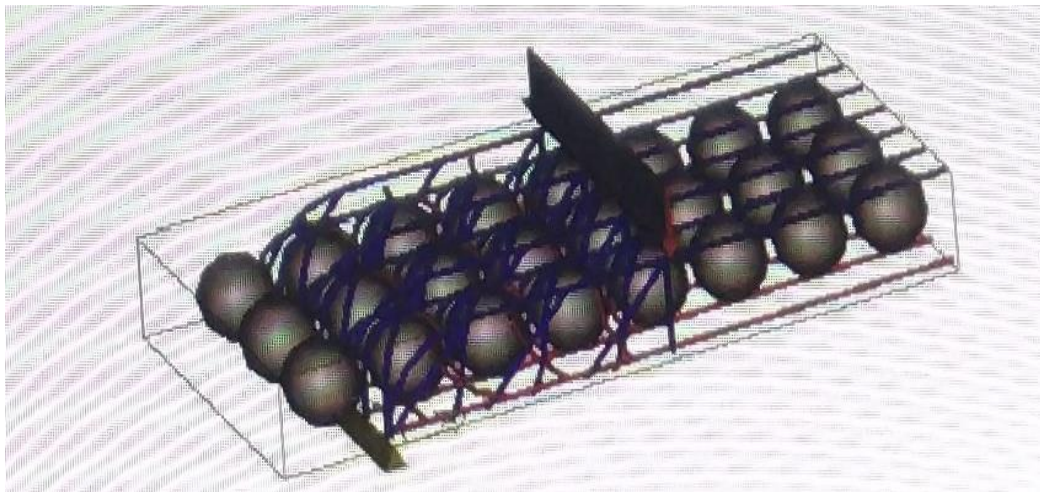
Gambar 10. Aliran Gaya 3D pada Pelat Beton Bertulang Berongga Bola (Aldejohann dan Schnellenbach, 2002)
