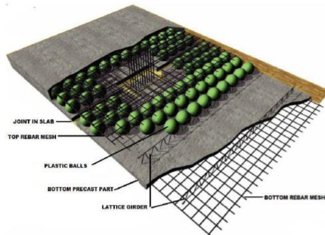
Gambar 7. Bubble Deck (Aldejohann dan Schnellenbach, 2003)
