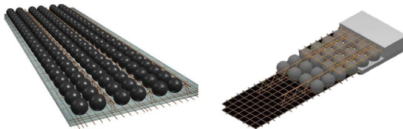
Gambar 8. Bubble Deck ( Betonwerk + Fertigteil Technik , 10/2005)
