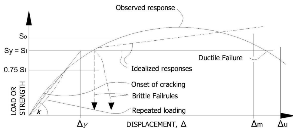
Gambar 2. Grafik Beton terhadap Lendutan Pelat Beton Getas dan Daktail
