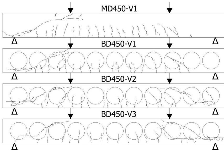
Gambar 15. Pola Retak Benda Uji Seri 1 (Aldejohann dan Schnellenbach, 2003)
