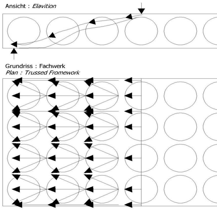
Gambar 9. Aliran Gaya pada Pelat Beton Bertulang Berongga Bola (Aldejohann dan Schnellenbach, 2002)
