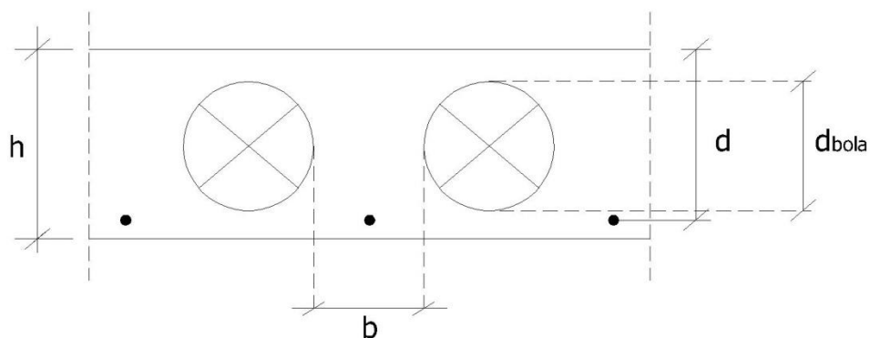
Gambar 12. Jarak Antar Bola (Aldejohann dan Schnellenbach, 2003)
