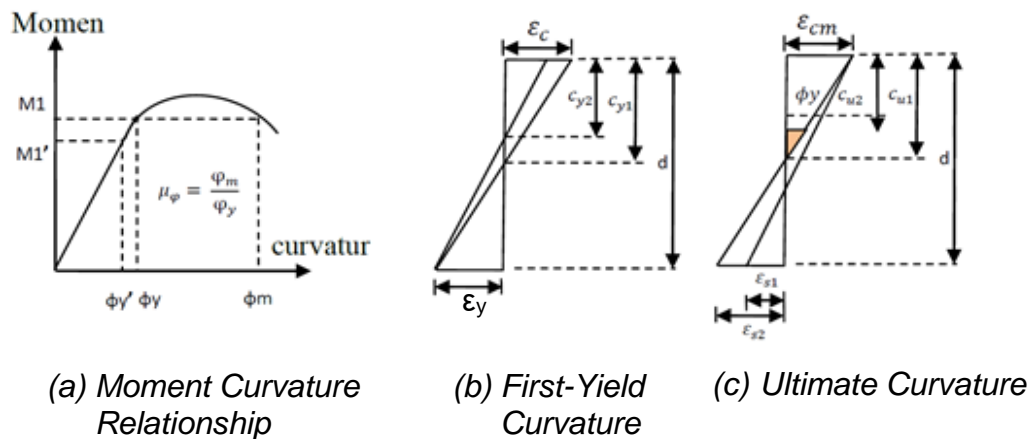
Gambar 4. Daktilitas Kelengkungan
