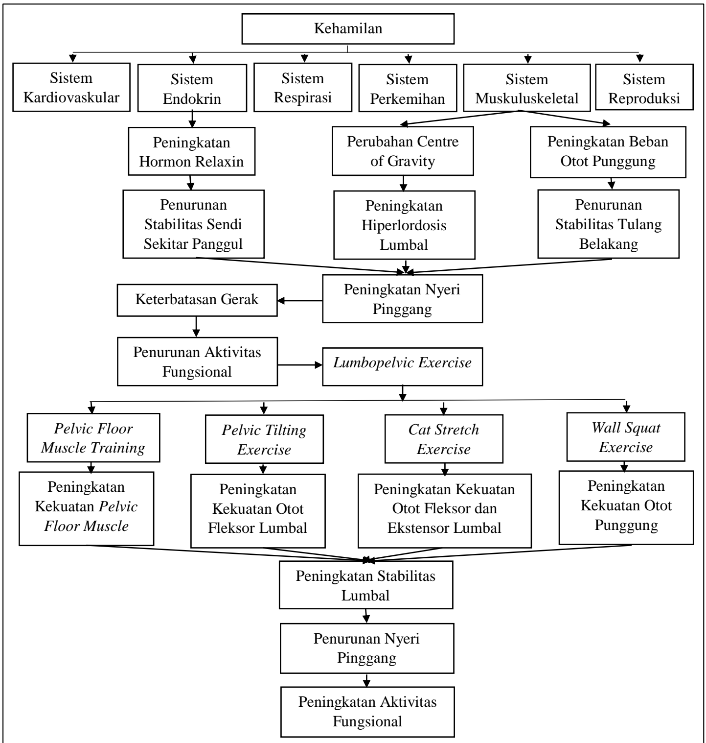
Gambar 2.9 Kerangka Teori
