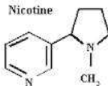
Gambar 1. Struktur Nikotin (27)
